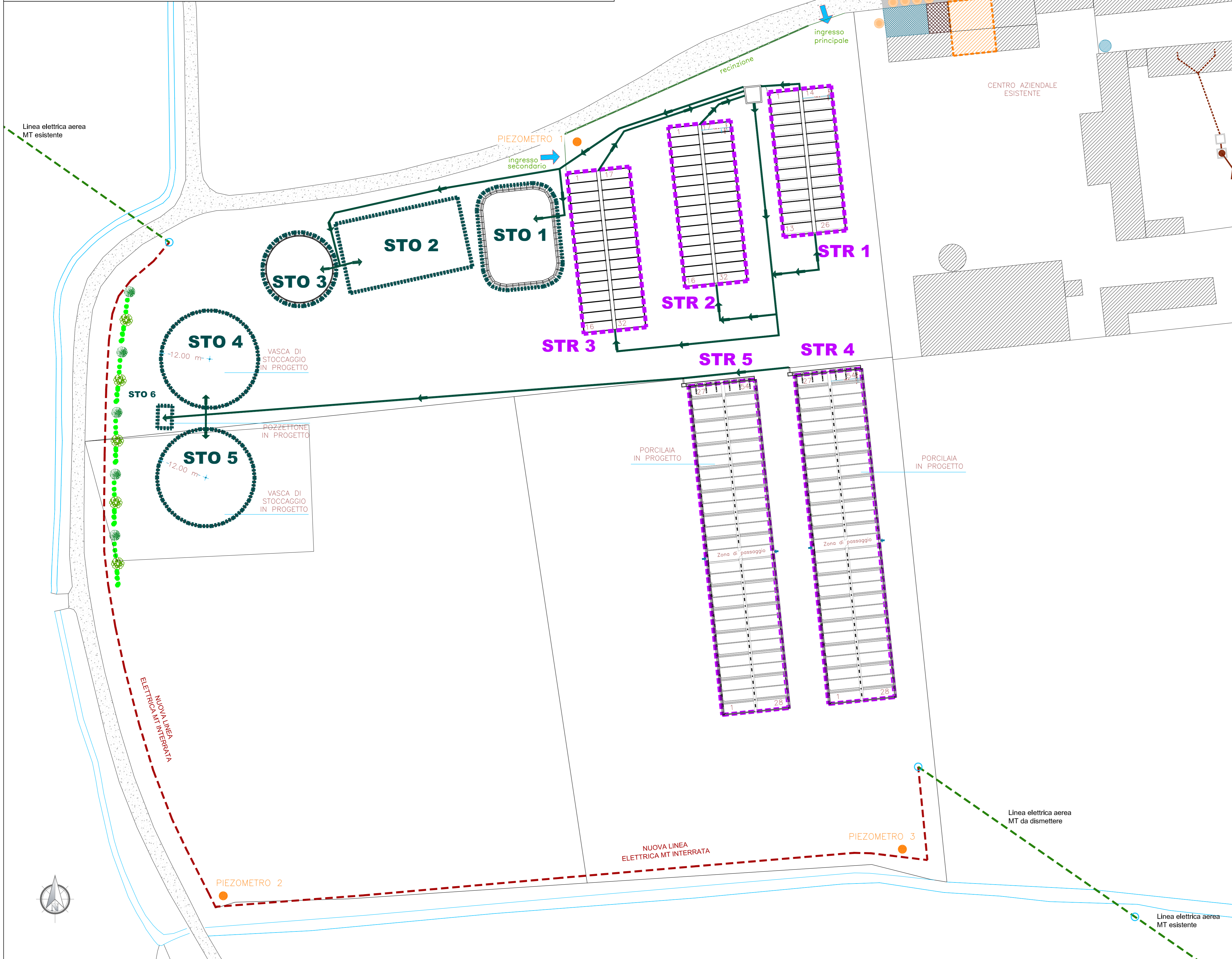
Planimetria generale di progetto - scala 1:500
