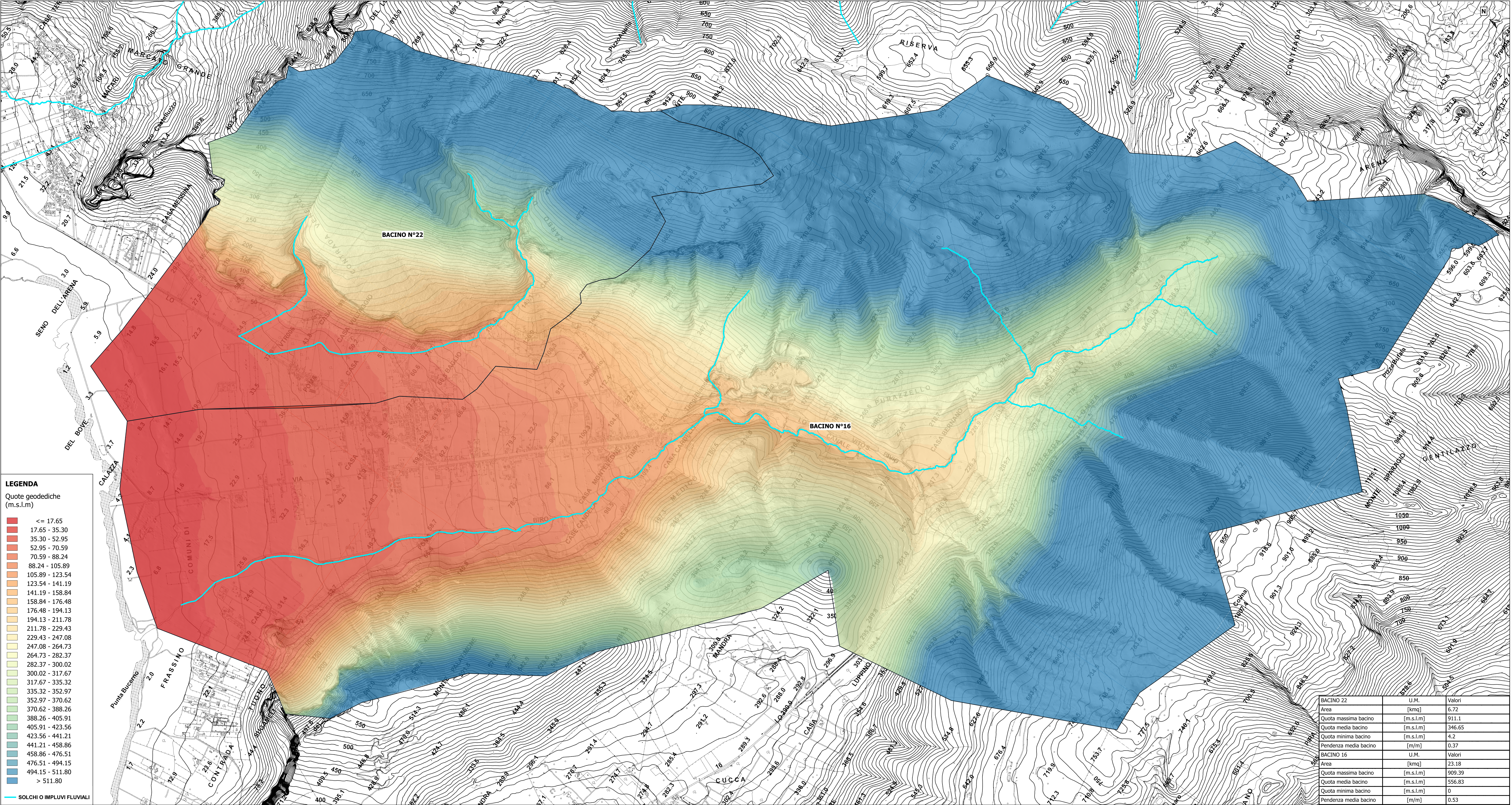
BACINO IDROGRAFICO SU CARTOGRAFIA TECNICA REGIONALE - Scala: 1:10.000 TEMATISMO: MODELLO DIGITALE DEL TERRENO - RISOLUZIONE 2 x 2 VISUALIZZAZIONE: BANDA SINGOLA FALSO COLORE Fonte: http://map.sitr.regione.sicilia.it/ArcGIS/services/DTM_2m/MapServer/WCSServer
