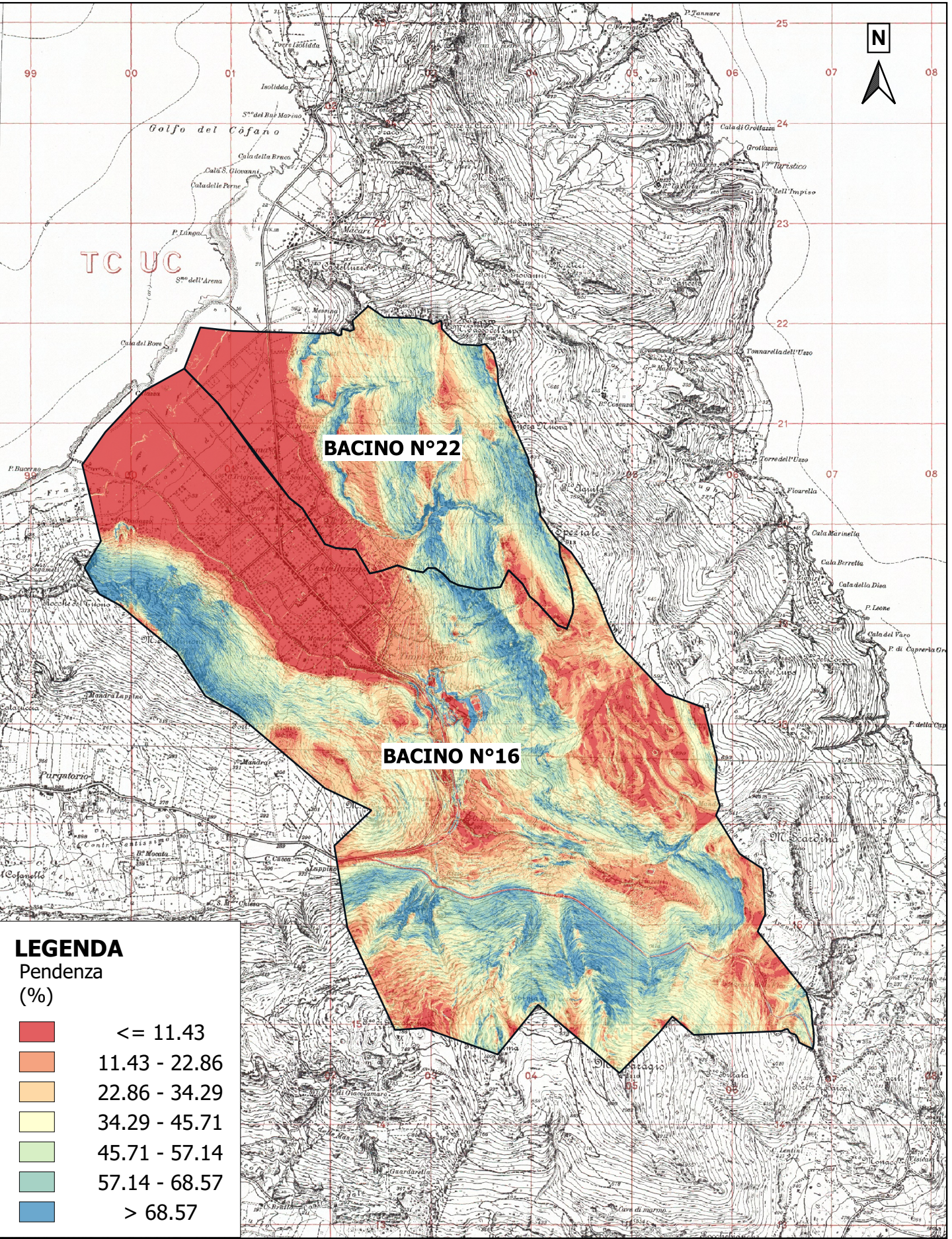
BACINO IDROGRAFICO SU CARTOGRAFIA TECNICA REGIONALE - Scala: 1:25.000 TEMATISMO: CARTA DELLE PENDENZE - RISOLUZIONE 2 x 2 VISUALIZZAZIONE: BANDA SINGOLA FALSO COLORE
